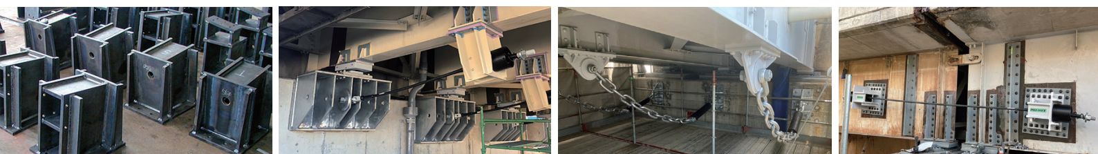
落橋防止システム
